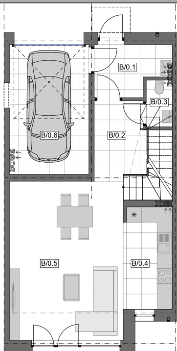
ZESTAWIENIE POWIERZCHNI - POZIOM 0
